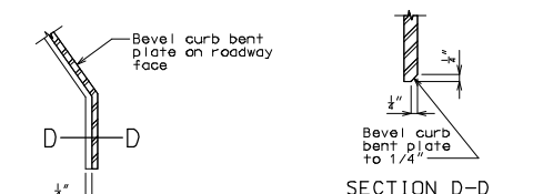
SECTION D-D
